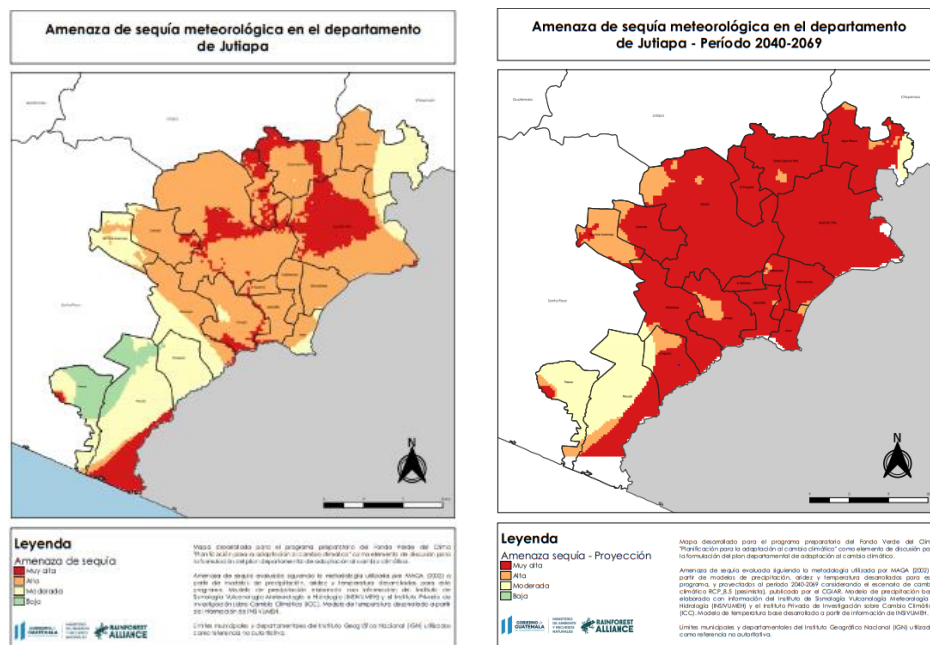
Figura 17. Mapa de Amenaza a sequía histórica y Mapa de Amenaza a sequía en escenario futuro (2050).
