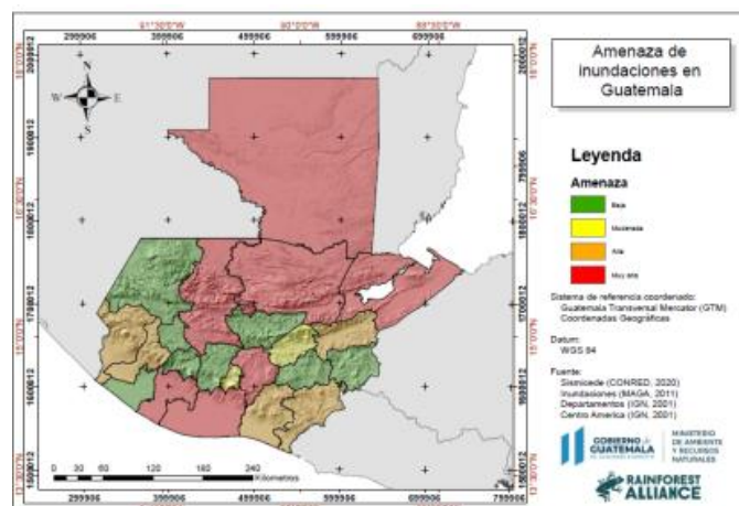
Figura 16. Mapa Amenaza de Inundaciones en Guatemala.
