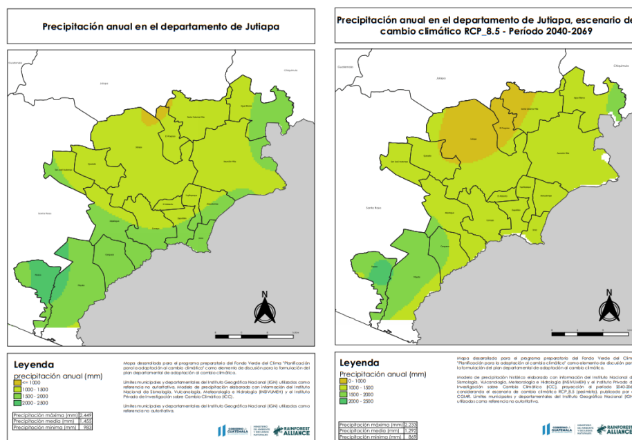
Figura 20. Mapa de Precipitación anual histórica y Mapa de Precipitación anual en escenario futuro (2050).
