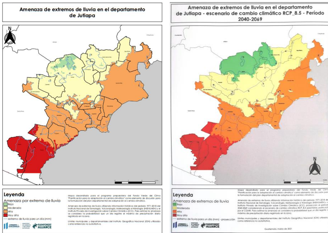
Figura 15. Mapa de Amenaza de extremos de lluvia histórica y Mapa de Amenaza de extremos de lluvia en escenario futuro (2050).
