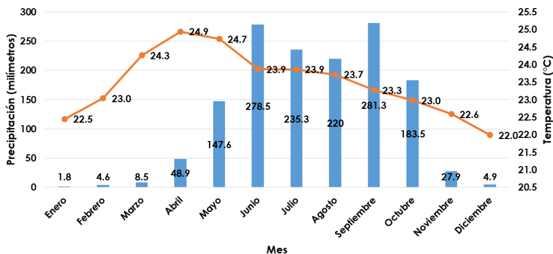
Figura 19. Climadiagrama del departamento de Jutiapa.
