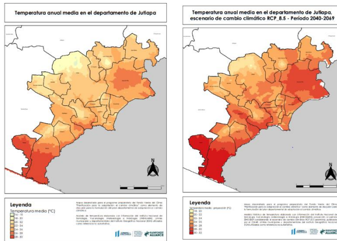
Figura 21. Mapa Temperatura anual media histórica y Mapa de Temperatura anual media en escenario futuro (2050).
