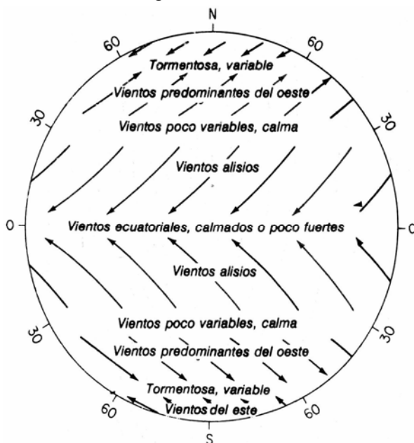
Gráfica No. 1 Circulación General de los Vientos
