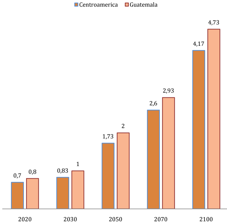
Centroamerica y Guatemala Comparación: Aumento de la temperatura Escenario A2 (Grados centigrados)
