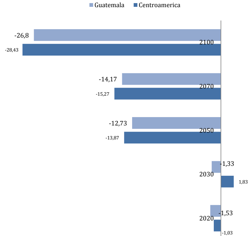
Centroamerica y Guatemala Comparación: Reducción % de precipitación, Escenario A2
